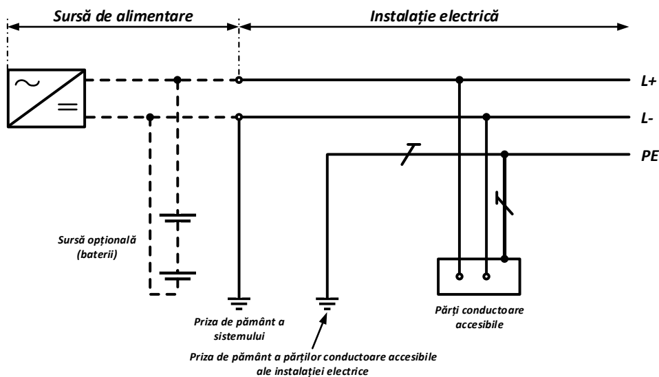
Figura 21. Schema sistemului TT cu conductorul de linie L- conectat la priza de pământ independentă electric de priza de pământ a părților conductoare accesibile ale instalației electrice
