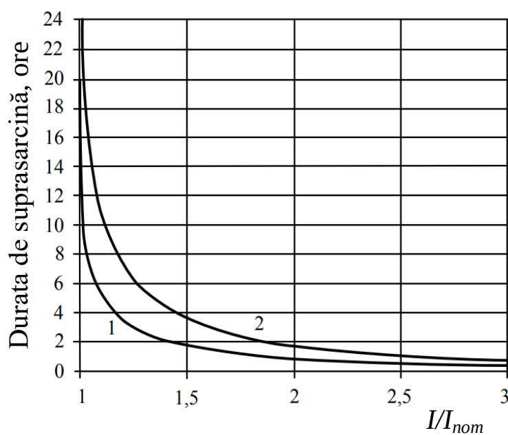
Figura 6. Durata admisibilă de suprasarcină a cablurilor cu trei conductoare cu izolație din polietilenă reticulată cu tensiunea mai mică de 35 kV în cazul conectării fără supraîncălzirea conductorului: 1 – pentru conductoare cu secțiunea de 35 mm 2 ; 2 – pentru conductoare cu secțiunea de 800 mm 2 .
