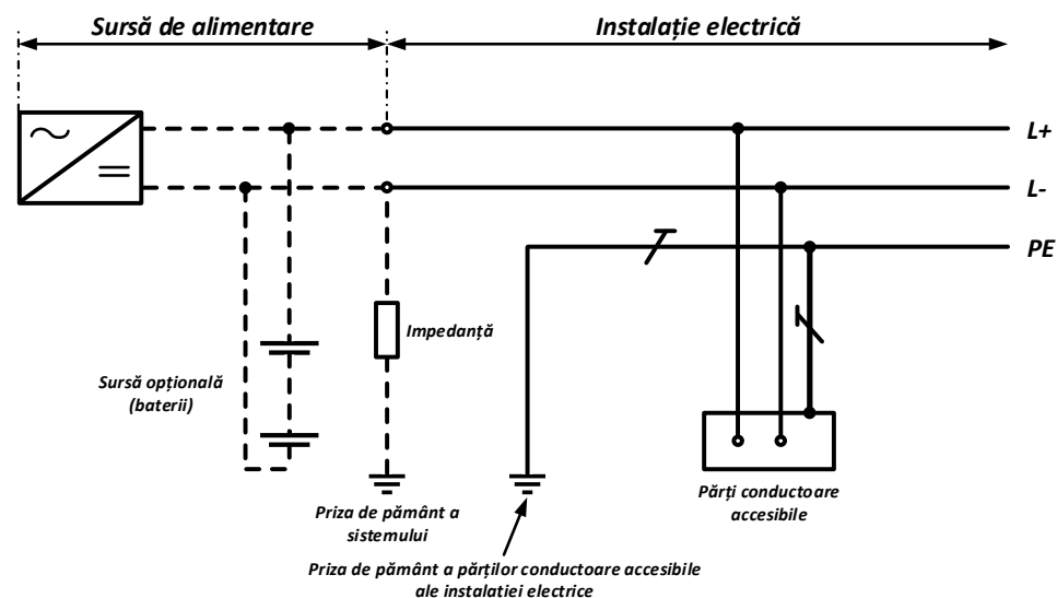
Figura 23. Schema sistemului IT cu conductorul de linie L- izolat sau legat la pământ printr-o impedanță de valoare mare. Părțile conductoare accesibile ale instalației electrice sunt legate la pământ
