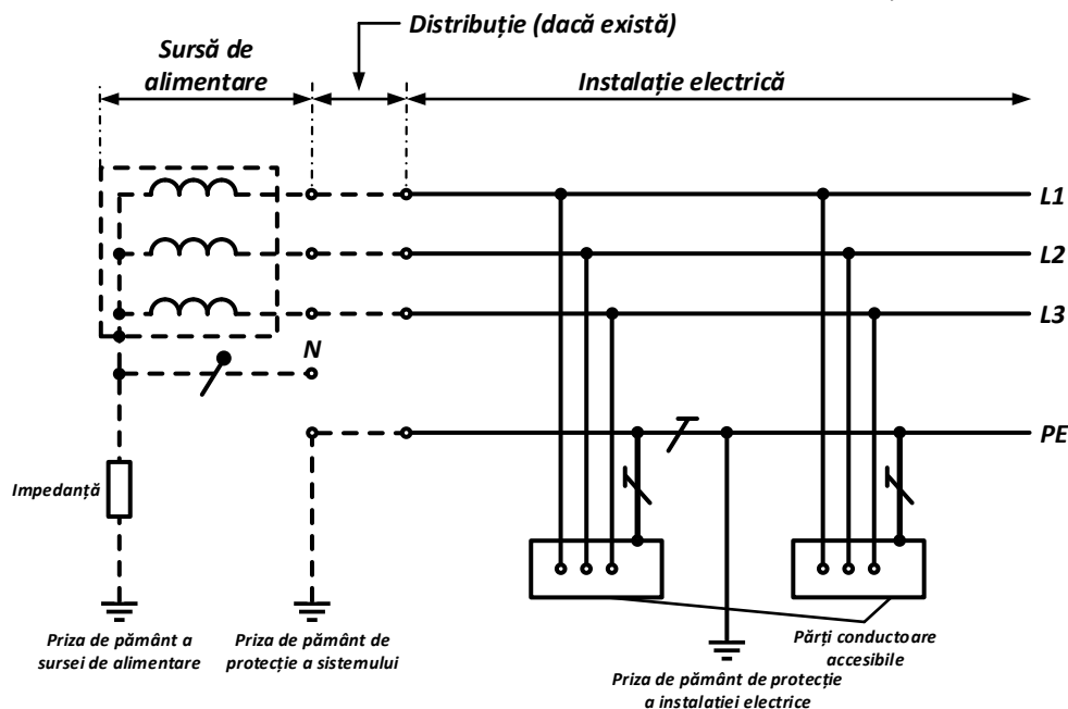
Figura 14. Schema sistemului IT cu toate părțile active ale sursei de alimentare izolate față de pământ sau o parte activă (punctul neutru) legată la pământ prin intermediul unei impedențe de valoare mare. Părțile conductoare accesibile ale instalației electrice sunt legate la pământ
