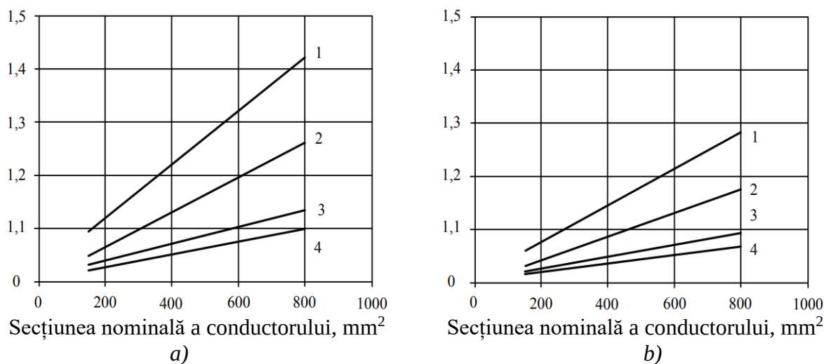
Figura 4. Coeficientul de corecție pentru schema de conectare a ecranelor cablurilor cu izolație din polietilenă reticulată cu tensiune mai mare de 110 kV:
