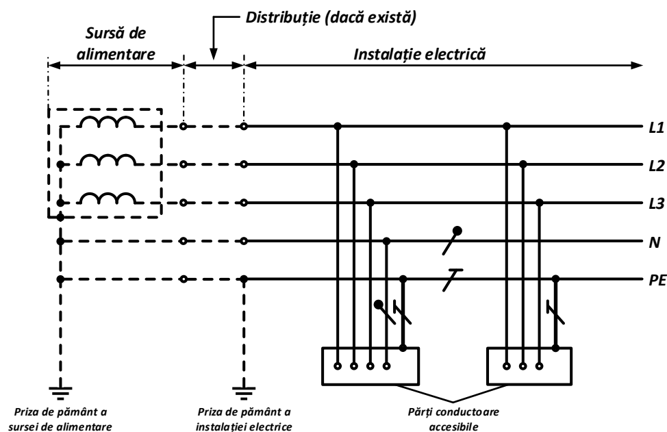
Figura 8. Schema sistemului TN-S cu conductor neutru N și conductor de protecție PE distincte pentru întregul sistem
