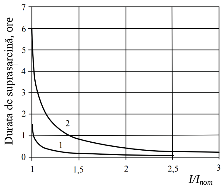
Figura 5. Durata admisibilă de suprasarcină a cablurilor monoconductoare cu izolație din polietilenă reticulată cu tensiunea mai mică de 35 kV în cazul conectării fără supraîncălzirea conductorului: 1 – pentru conductoare cu secțiunea de 35 mm 2 ; 2 – pentru conductoare cu secțiunea de 800 mm 2 .
