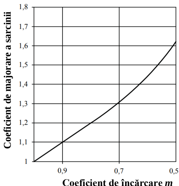
Figura 1. Coeficientul de corecție pentru coeficientul de încărcare m al cablurilor cu izolație din polietilenă reticulată cu tensiunea mai mică de 35 kV
