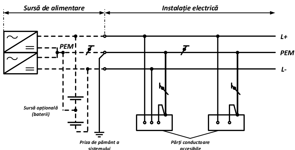
Figura 18. Schema sistemului TN-C cu funcțiile conductorului de punct median M legat la pământ și ale conductorului de protecție PE combinate într-un singur conductor PEM pentru întregul sistem
