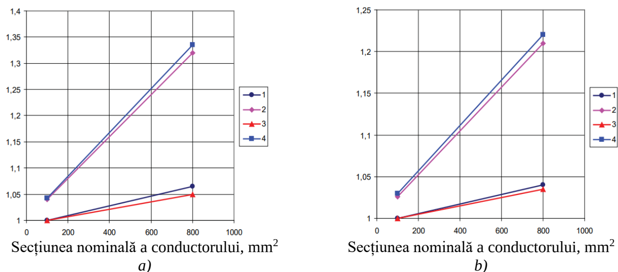
Figura 3. Coeficientul de corecție pentru schema de conectare a ecranelor cablurilor cu izolație din polietilenă reticulată cu tensiune mai mică de 35 kV:
