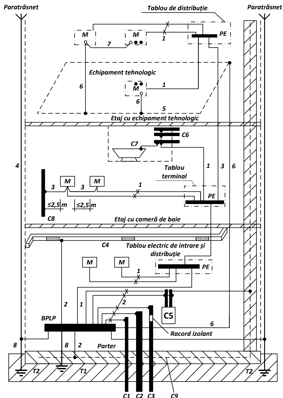
Figura 26. Sistemul de echipotențializare în clădiri:
